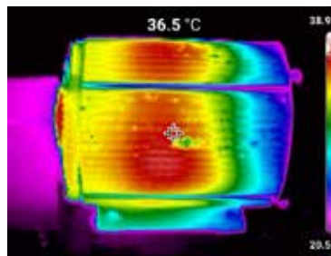
Infraröd bild av motor från Fluke TiS55+-värmekamera
